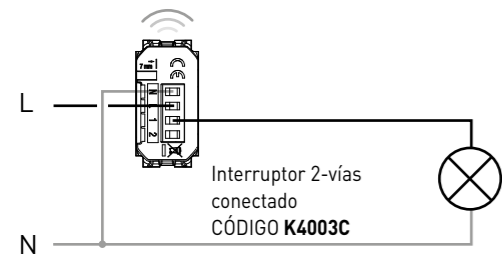
Diagrama de cableado - interruptor
