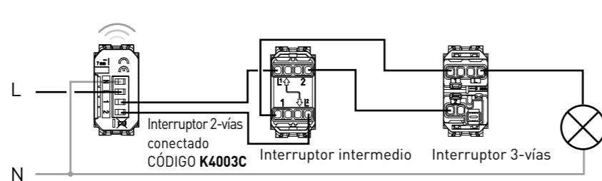
Diagrama de cableado - Invertido o redirigido
